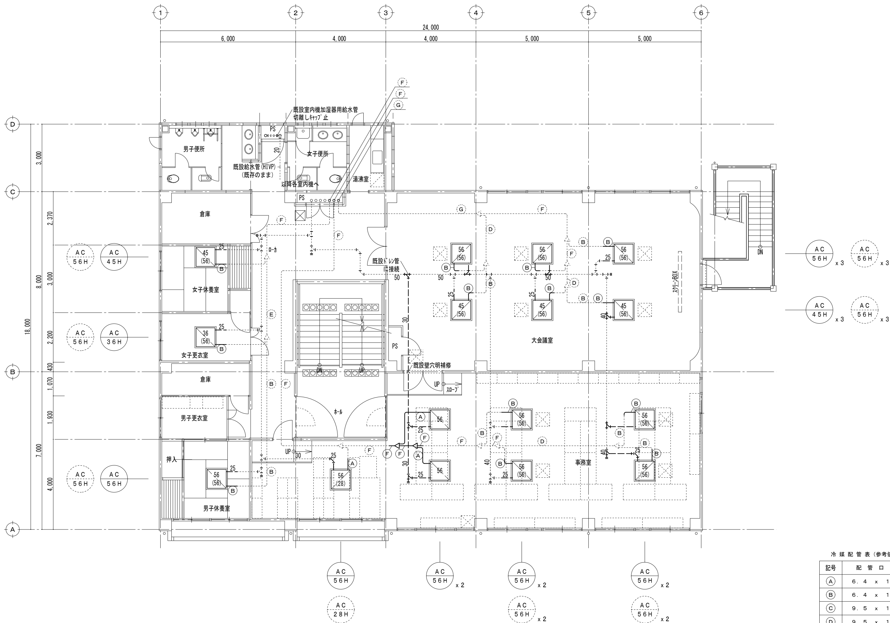
3階平面図 SC=1/100
